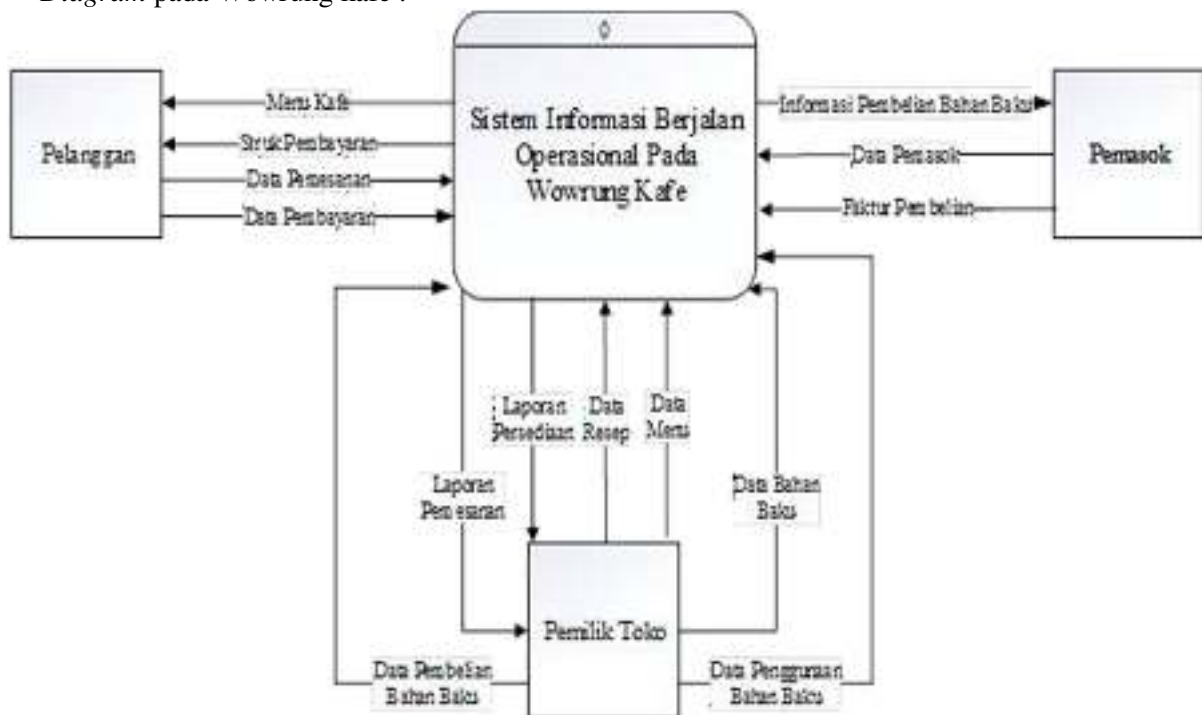
Gambar 4. DFD Konteks Sistem Informasi Berjalan Operasional di Wowrung Kafe
