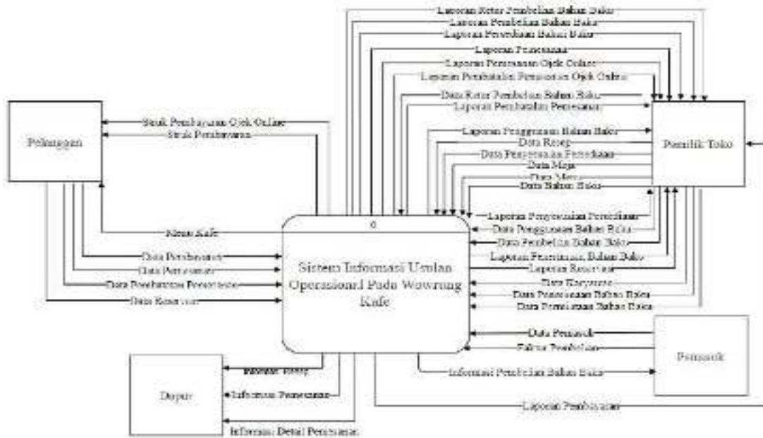
Gambar 6. DFD Konteks Sistem Usulan
