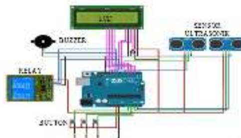
Gambar 8. Rangkaian Keseluruhan
