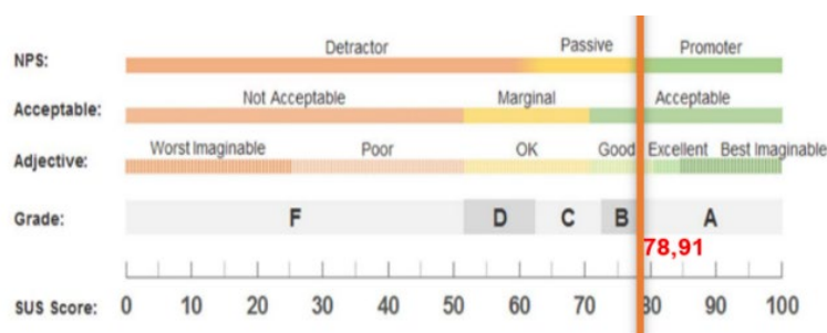
Gambar 18. Skor SUS
