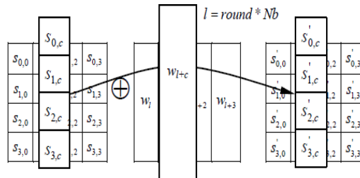
Gambar 5 Ilustrasi Transformasi AddRoundKey.[6]
