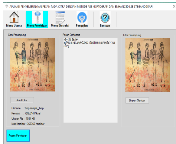
Gambar 10. Proses Penyisipan.
