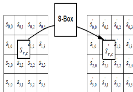
Gambar 6 Transformasi SubByte[6].
