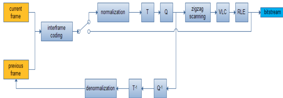
Gambar 2 Skema Encoder
