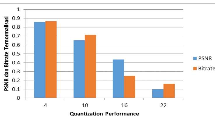
Gambar 6 Grafik Penurunan PSNR dan Bitrate sesuai Nilai QP yang diberikan
