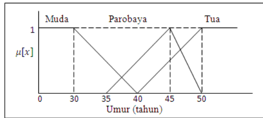
Gambar 4. Fungsi Keanggotaan
