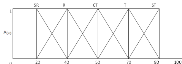
Gambar 9. Grafik Bobot
