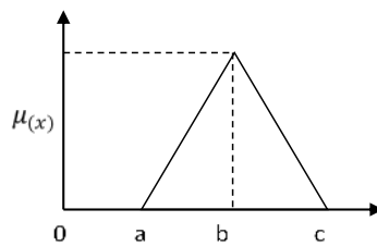
Gambar 10. Kurva Segitiga
