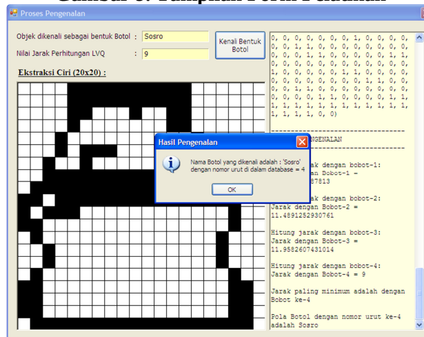
Gambar 10. Tampilan Hasil Proses Pengenalan
