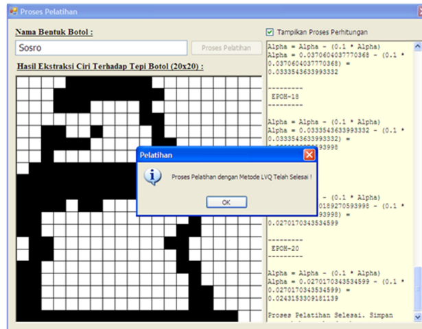
Gambar 9. Tampilan Form Pelatihan
