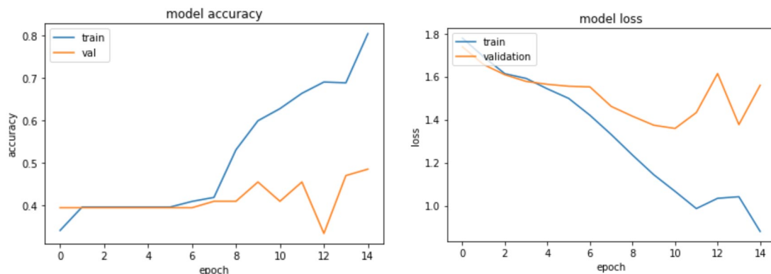
Gambar 7. Akurasi Model
