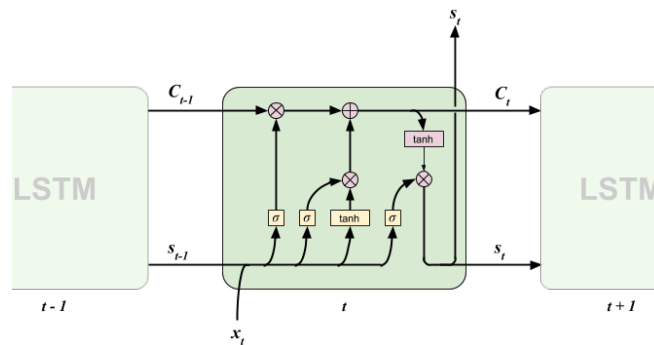
Gambar 1. Arsitektur LSTM
