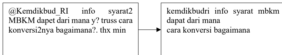
Gambar 3. Data latih 1 sebelum dan sesudah pre-processing
